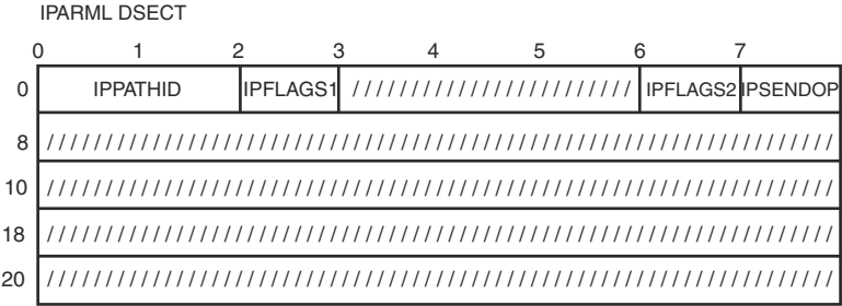
Figure 41. APPCVM SENDCNFD Input Parameter List
